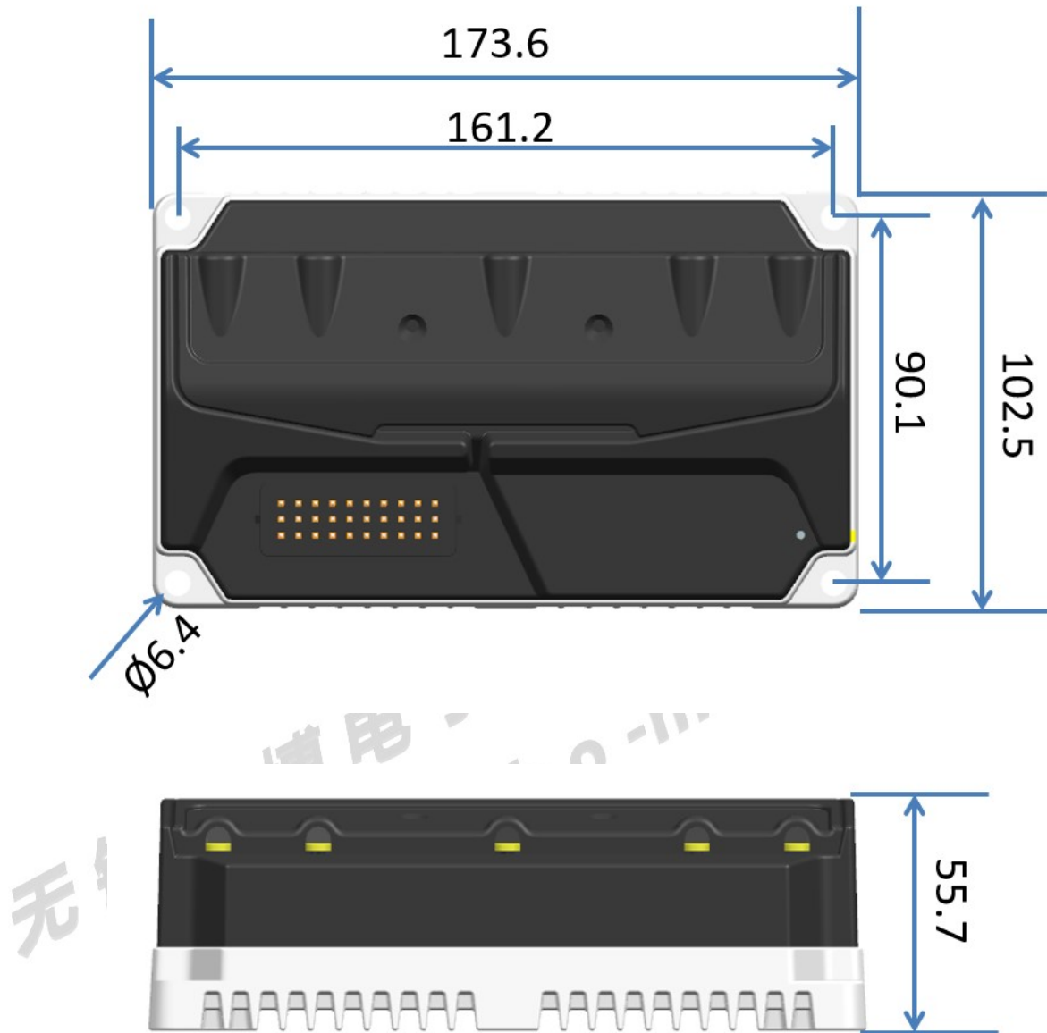
LBMC EK5XE 外形示意图
